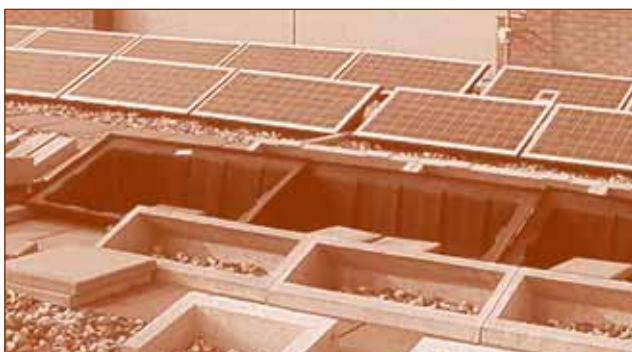
Verschillende standaardsystemen in beton of kunststof voor opstelling van PV-modules op een plat dak (Ecofys)
